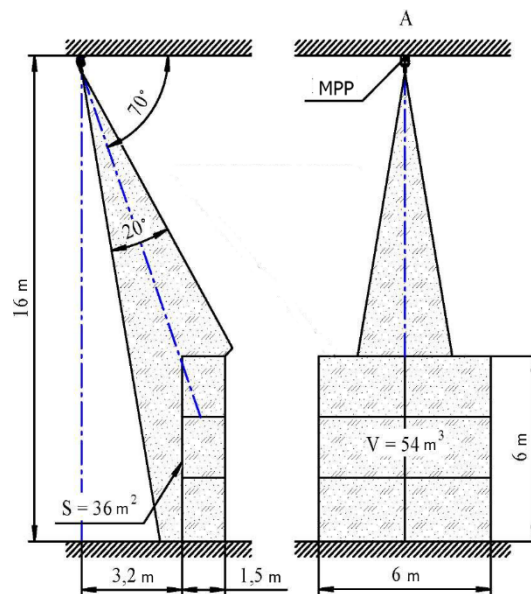
Bild 6. Installation MPH für Regalschutz bei Bränden Klasse A.
