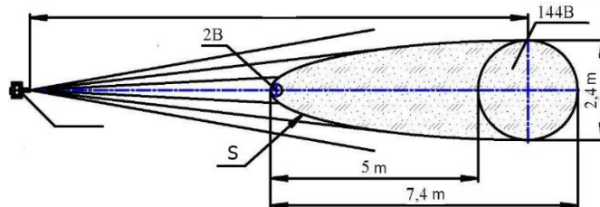
Fig. 7. Instalación MPH a una altura de 1 m con un ángulo de eje de 3^\circ
