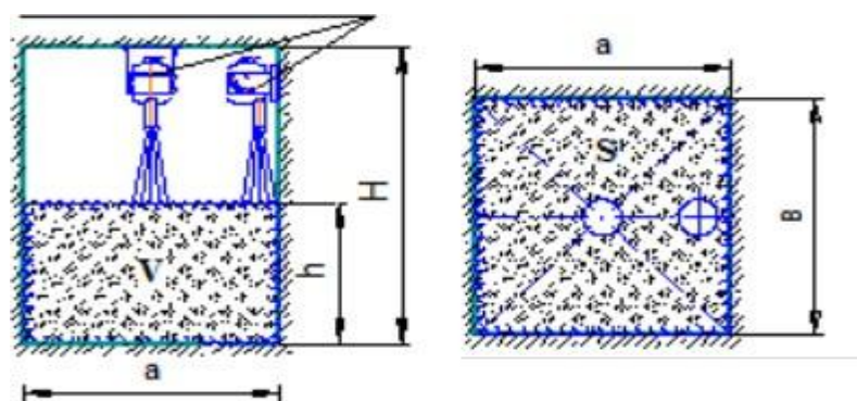
Fig 5. MPH instalado en ángulo, para protección local de objetos con áreas de sombra para incendios de clase A
