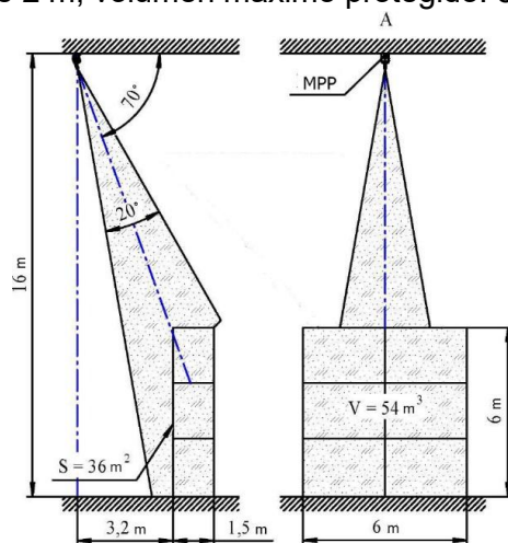
Fig. 6. Instalación de MPH para protección de estanterías en incendios de clase A.
