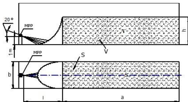
Fig. 4. El MPH instalado en la interior o conducto a una altura de 1 m del suelo con un ángulo de eje de 20 grados y el inserto del atomizador apuntando hacia abajo.
