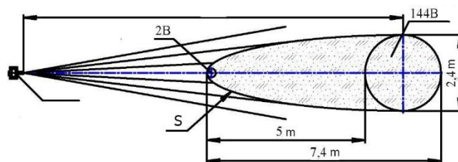
Bild 7. Installation MPH in Höhe 1m mit Achsenwinkel 3^\circ
